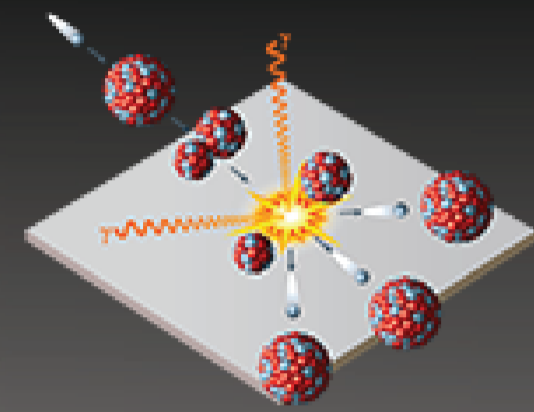
Gamma ray / Rayon gamma
