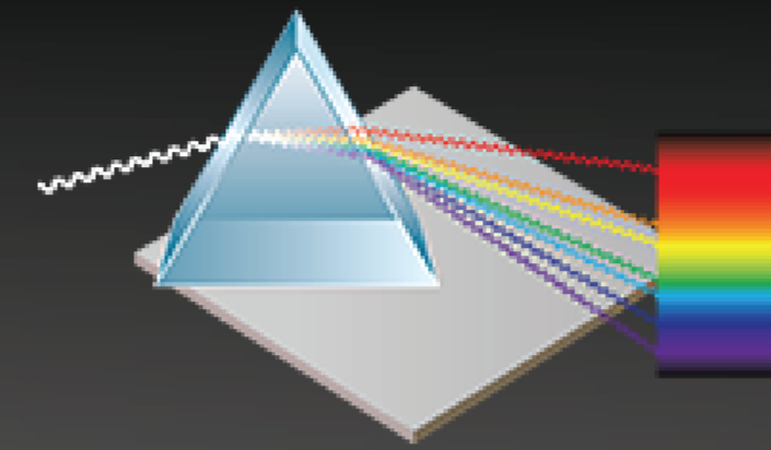
Visible light / Lumière visible
