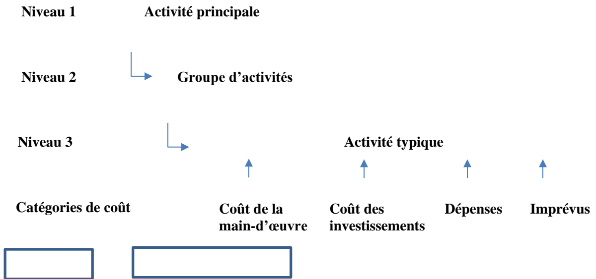
Figure 1 : Structure hiérarchique des coûts selon l'International Structure for Decommissioning Costing [5]
