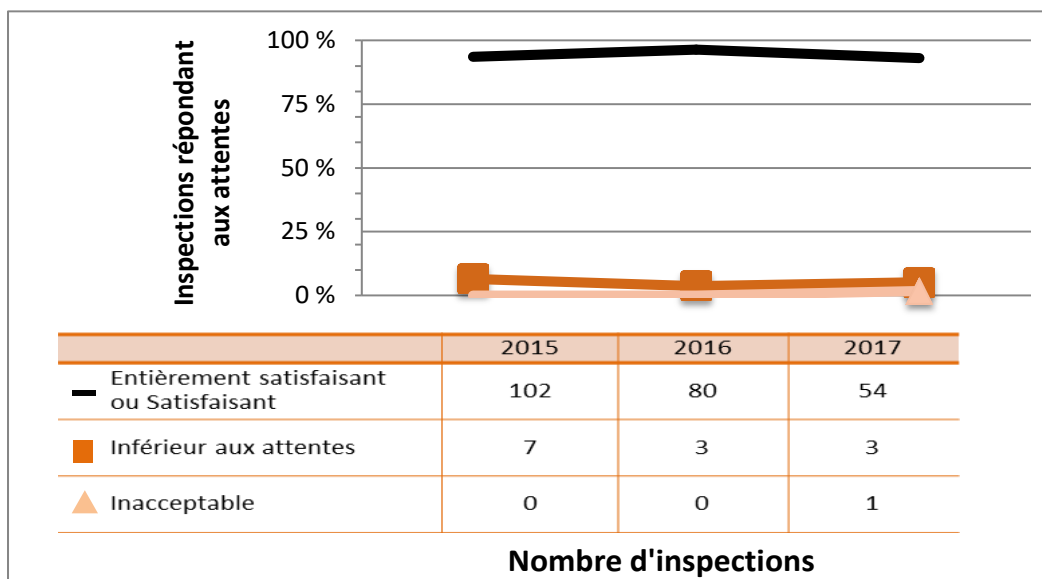
Figure 52 : Rendement du secteur commercial – cotes d'inspection pour le DSR Système de gestion de 2015 à 2017
