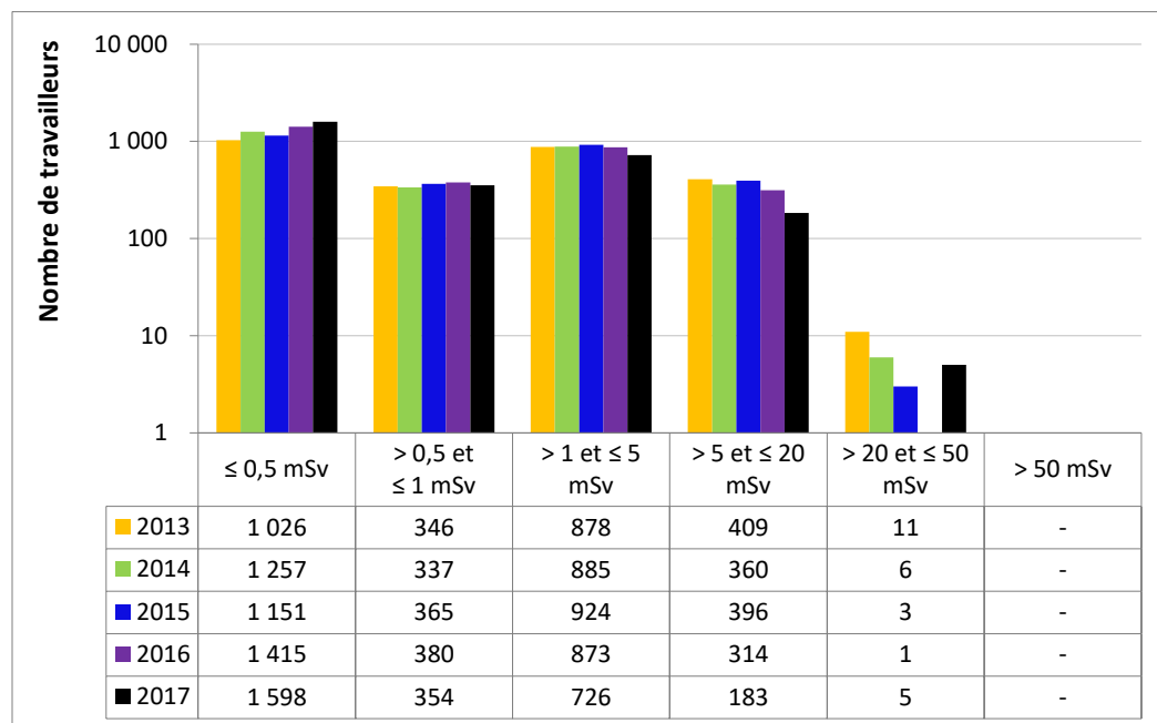
Figure 30 : Rendement du sous-secteur de la gammagraphie industrielle – doses efficaces annuelles reçues par les TSN de 2013 à 2017
