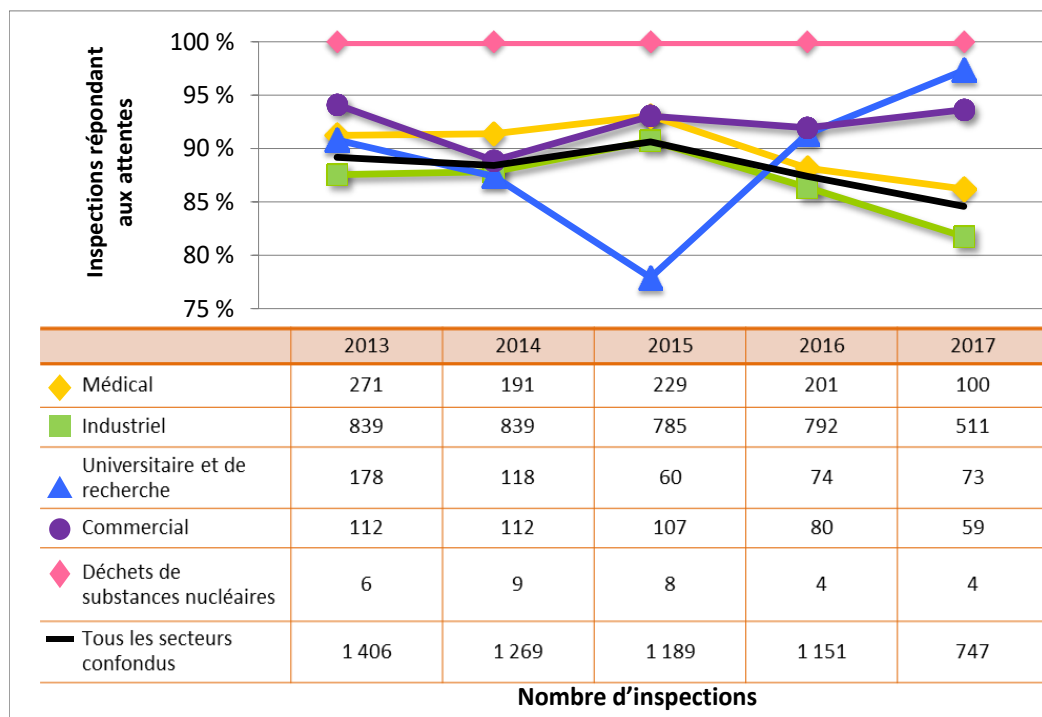
Figure 7 : Comparaison secteur par secteur des cotes d'inspection atteignant ou dépassant les attentes pour le DSR Conduite de l'exploitation, 2013 à 2017
