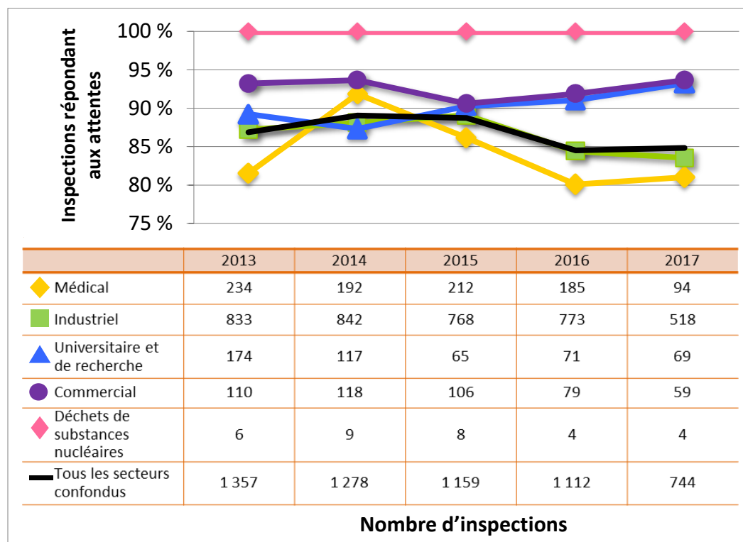
Figure 10 : Comparaison secteur par secteur des cotes d'inspection atteignant ou dépassant les attentes pour le DSR Radioprotection, 2013 à 2017
