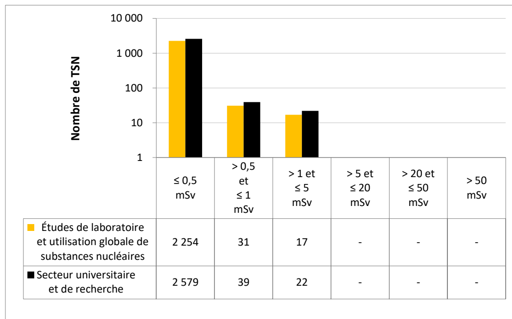
Figure 40 : Comparaison du rendement du secteur universitaire et de la recherche – doses efficaces annuelles reçues par les TSN en 2017
