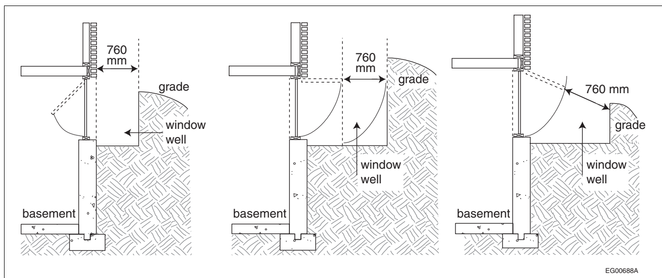
Figure A-9.9.10.1.(3)
