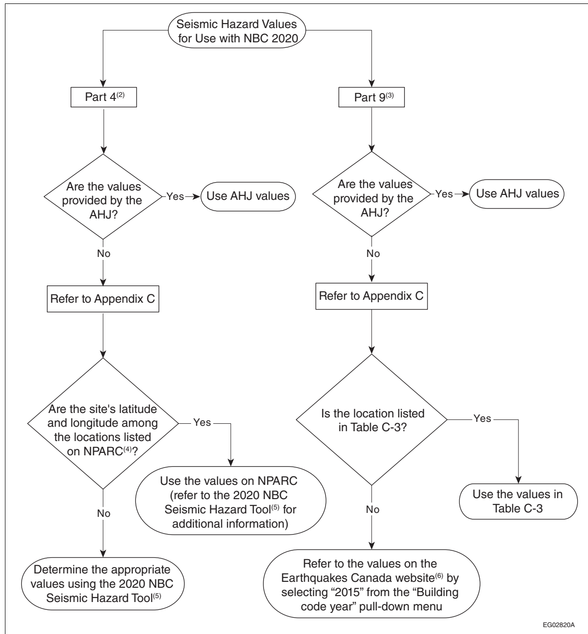
Figure A-1.1.3.1.(4)
