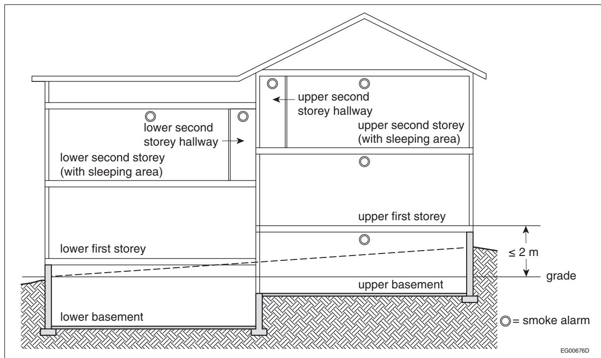
Figure A-9.10.19.3.(1)
