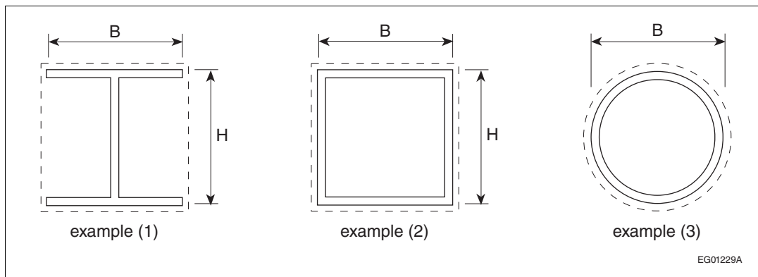
Figure D-2.6.4.-A
