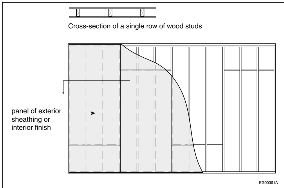
Figure A-9.10.3.1-F
