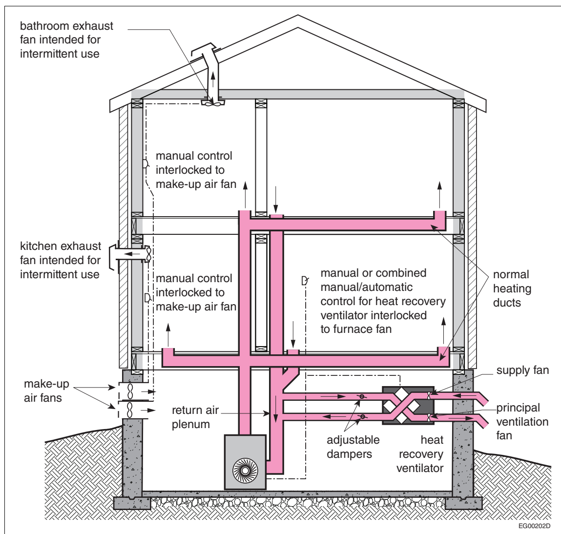
Figure A-9.32.3.3.-B
