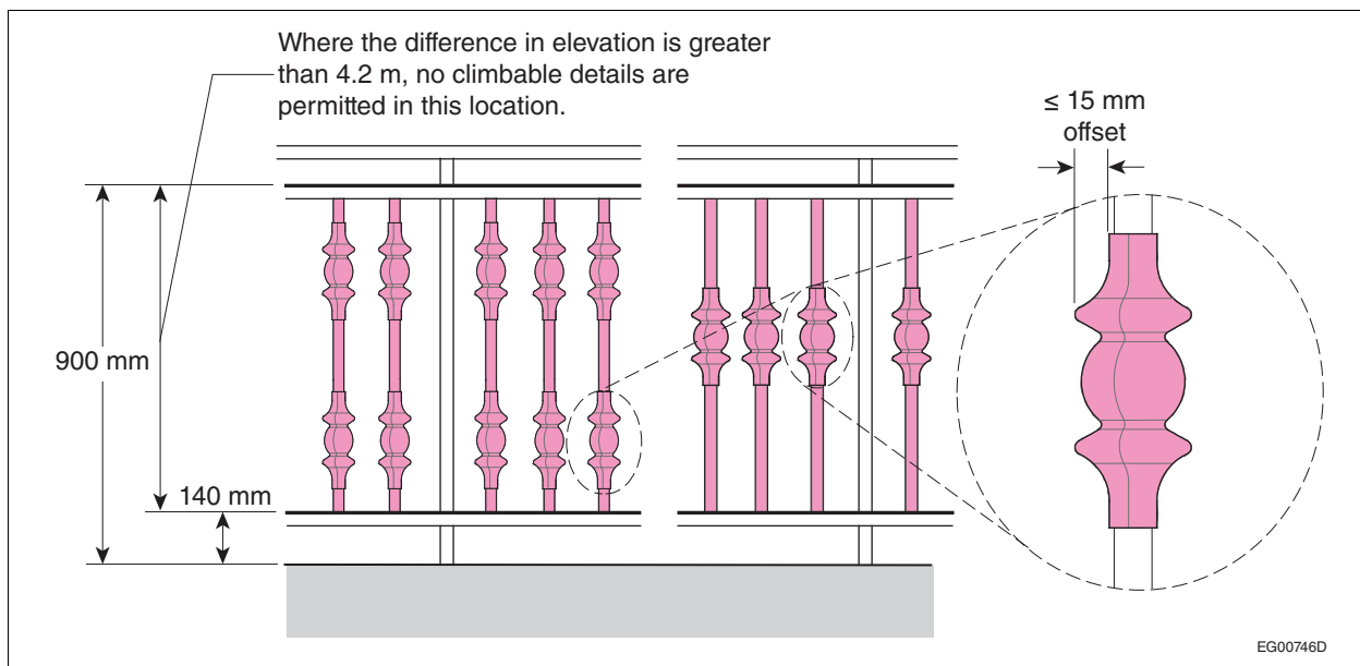
Figure A-9.8.8.6.(1)-B
