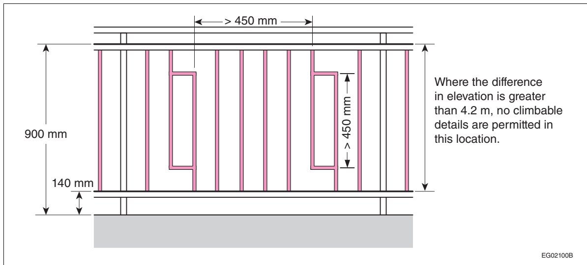
Figure A-9.8.8.6.(1)-A
