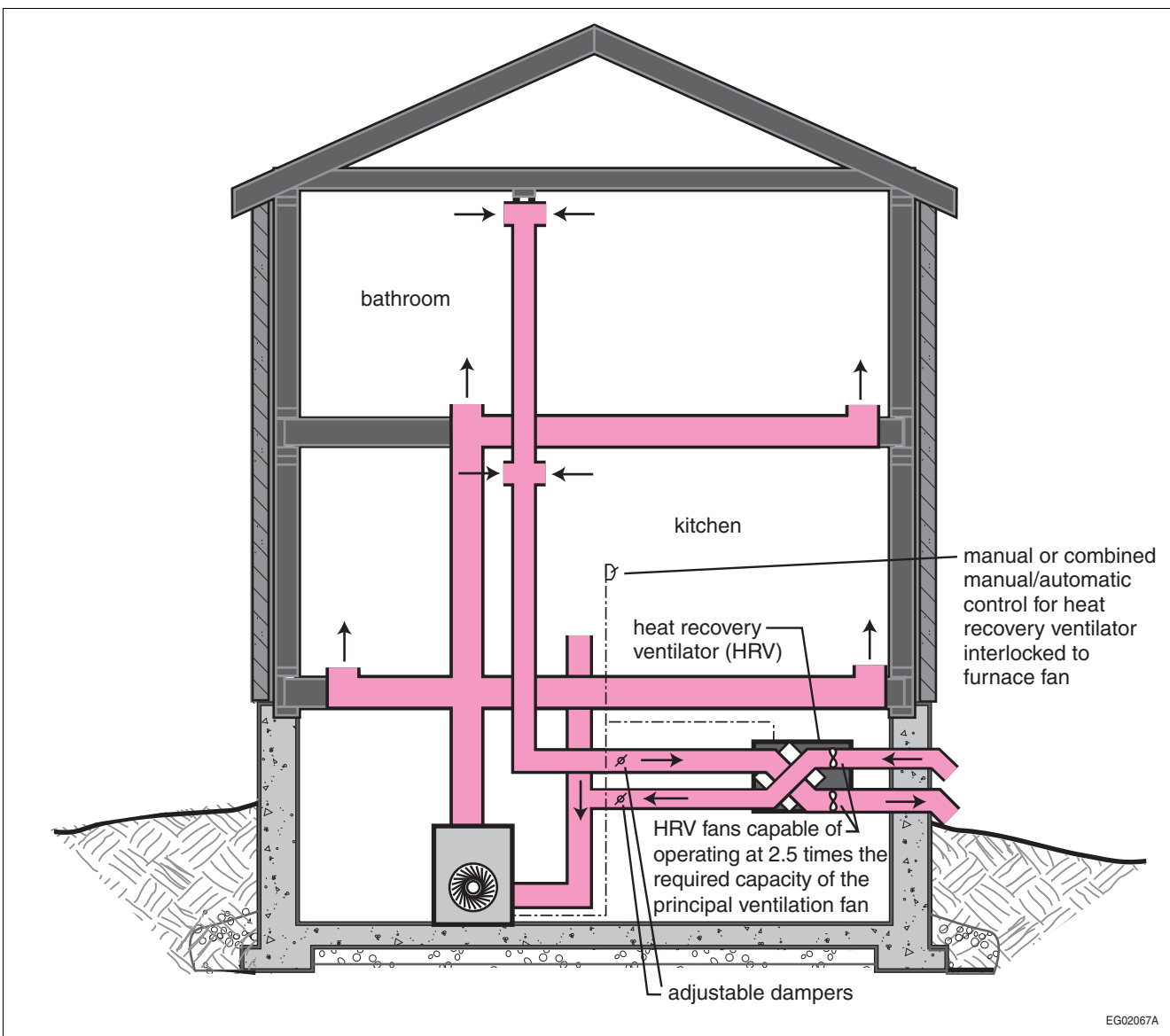
Figure A-9.32.3.3.-F
