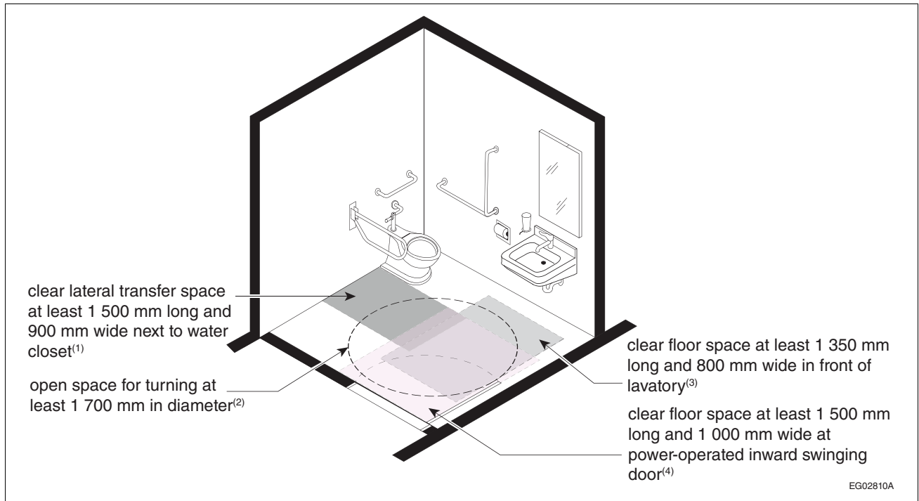
Figure A-3.8.3.13.-B
