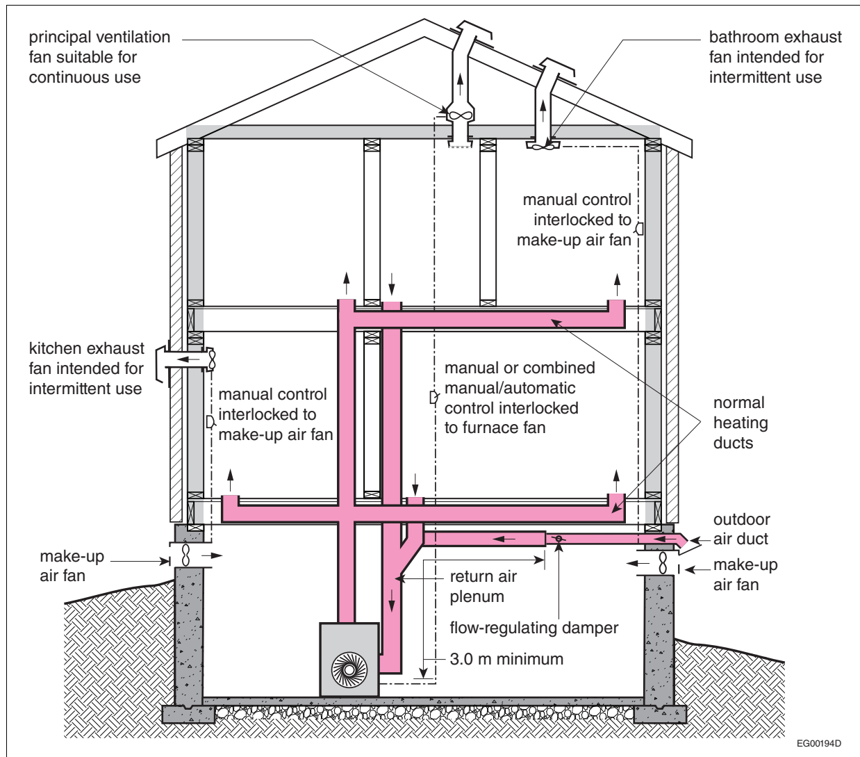
Figure A-9.32.3.3.-A
