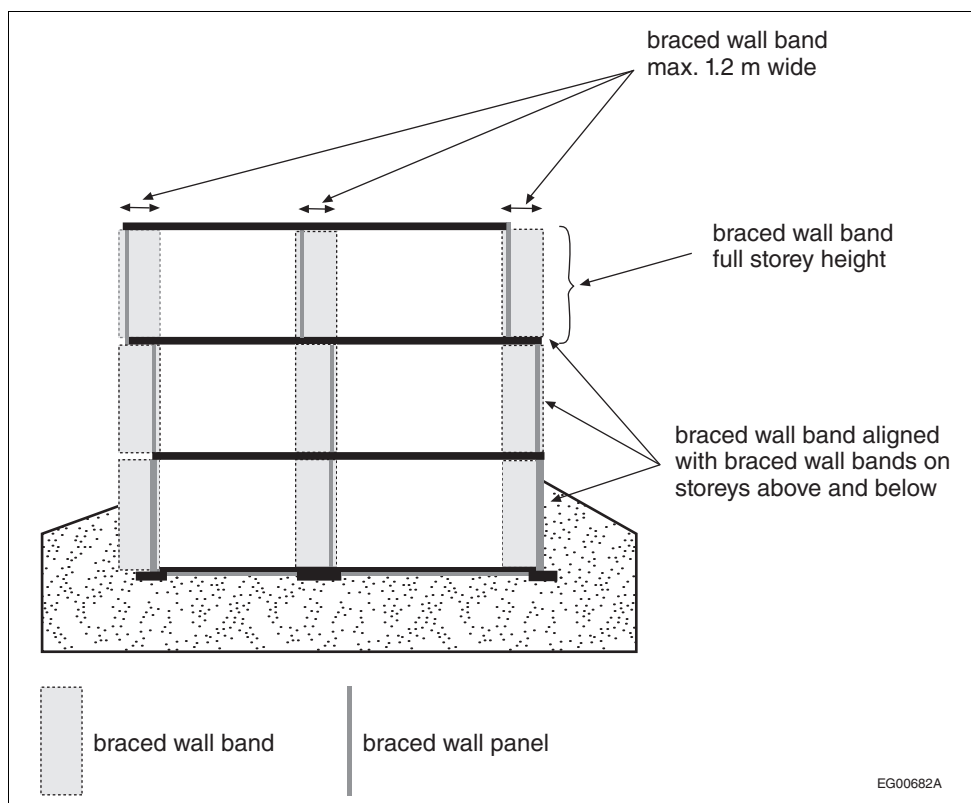
Figure A-9.23.13.4.-A
